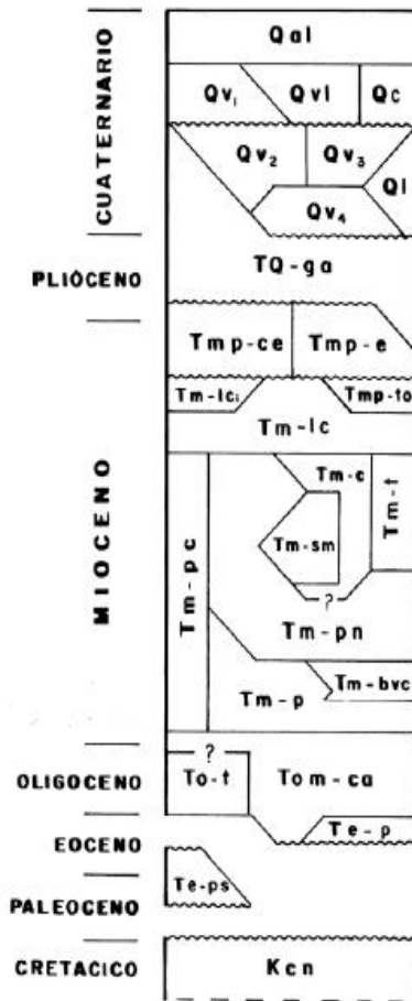
Fig. 2: Columna estratigráfica. Complejo de Nicoya (Kcn), Fm. Punta Serrucho (Te-ps), Fm. Parritilla (Te-p), Fm. Carraigres (Tom-ca), Miembro Tranquerillas (To-t), Fm. Punta Carballo (Tm-pc), Fm. Pacacua (Tm-p), Brechas verdes Coyolar (Tm-bvc), Fm. Peña Negra (Tm-pn), Fm. San Miguel (Tm-sm), Fm. Coris (Tm-c), Fm. Turrúcares (Tm-t), Fm. La Cruz (Tm-ic), Depósitos Parálidos de Fm. La Cruz (Tm-lci), Tobitas Ococa (Tmp-to), Intrusivo de Escazú (Tmp-e), Comubianitas de Escazú (Tmp-ce), Fm. Grifo Alto (TQ-ga), Fm. Lavas intracañón (Qv4), Fm. Depósitos de Avalancha Ardiente (Qv3), Fm. Orotina (Qv2), Fm. Barva (Qv1), Depósitos lacustres (Ql), Calizas deslizadas (Qc). Lahares y cenizas (Qv1), Depósitos aluviales y coluviales recientes (Qal). (Figura 2: Fuente Denyer y Arias, 1991)
